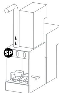
Horno atmosférico (tiro natural)
