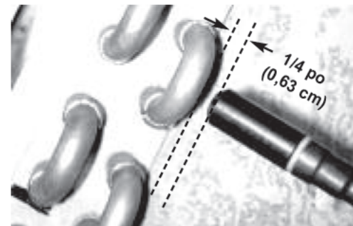
Serpentin en A testé dans un évaporateur par le SRL2, à 1/4 po (0,63 cm) du tuyau.
